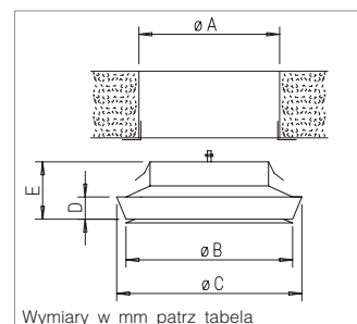
Wymiary w mm patrz tabela
